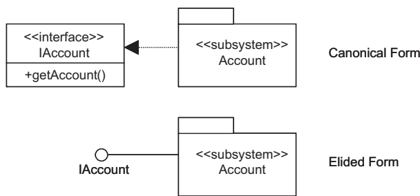
Fig. 2. UML component.
